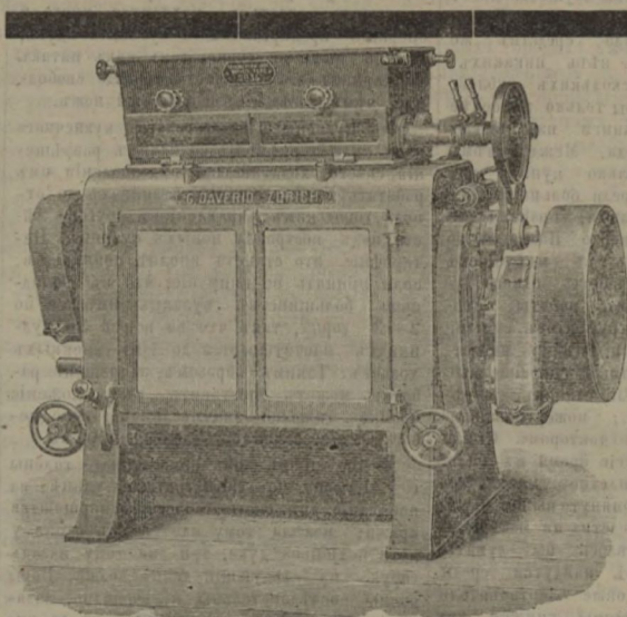
Трехвалвный станокъ новѣйшей онструціи.
