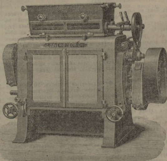
Трехвальцовый станокъ новѣйшей конструкціи.
