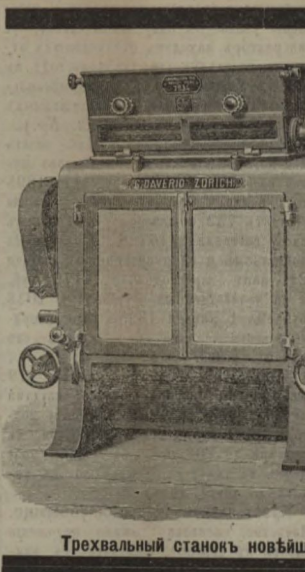
Трехвалный станокъ новѣйшей конструкціи.
