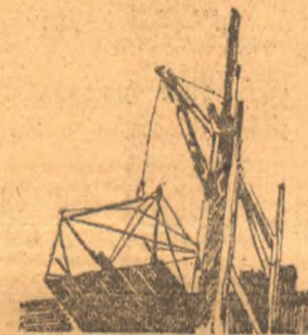
На стройке дома железнодорожников. Электрическая подъемная машина поднимает наверх до 10 тыс. кирпичей в день.
