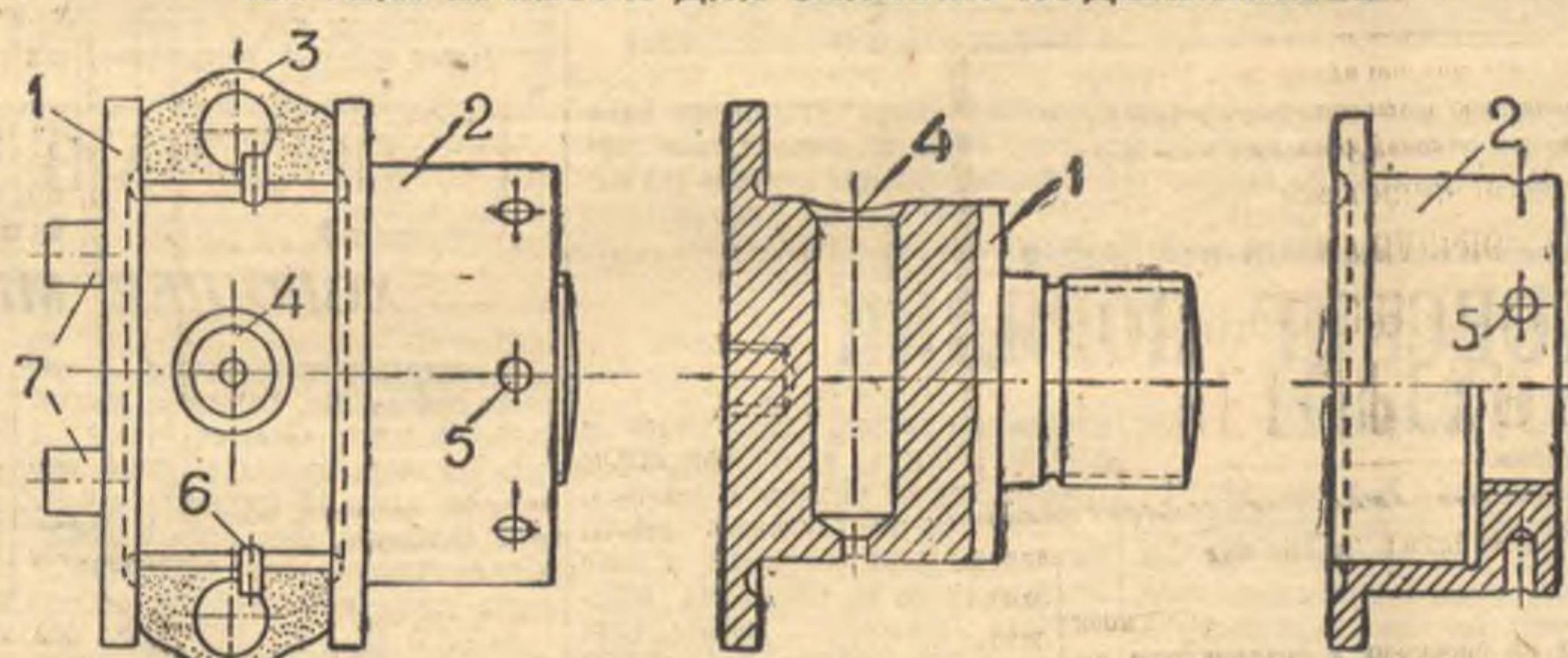
ЧЕРТЕЖ ПРИБОРА ДЛЯ ЗАЛИВКИ ПОДШИПНИКОВ
