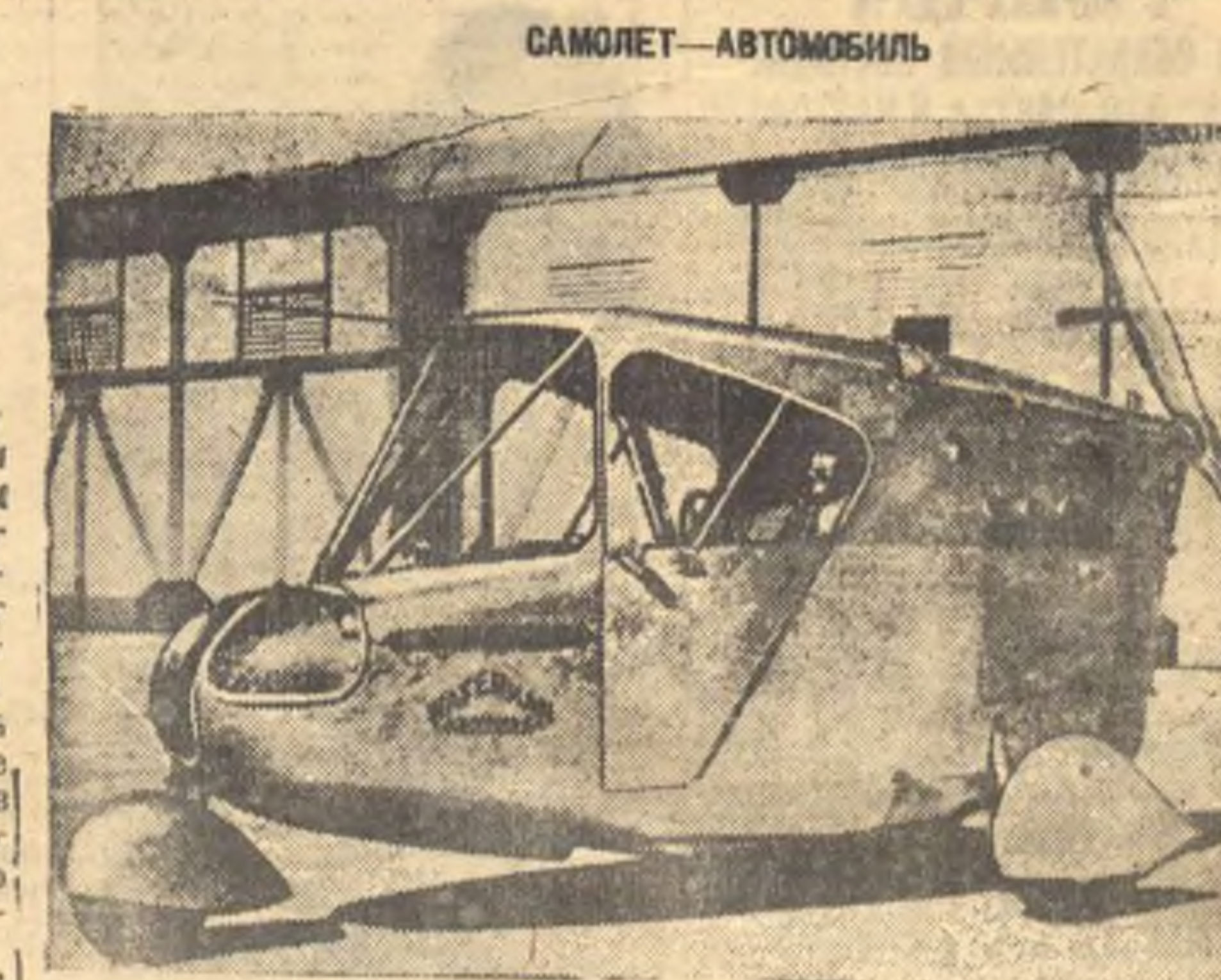
Американский конструктор В. Уотерман сконструировал оригинальный самолет, который может быть после приземления и снятия крыльев использован как автомобиль. Самолет снабжен шестигидравлическим мотором «Студебекер». Скорость его в воздухе до 200 км. в час, на земле — до 80 км. в час. На снимке: самолет-автомобиль после снятия с него крыльев на аэродроме в Санта-Моника (штат Калифорния). (Совдепото).
