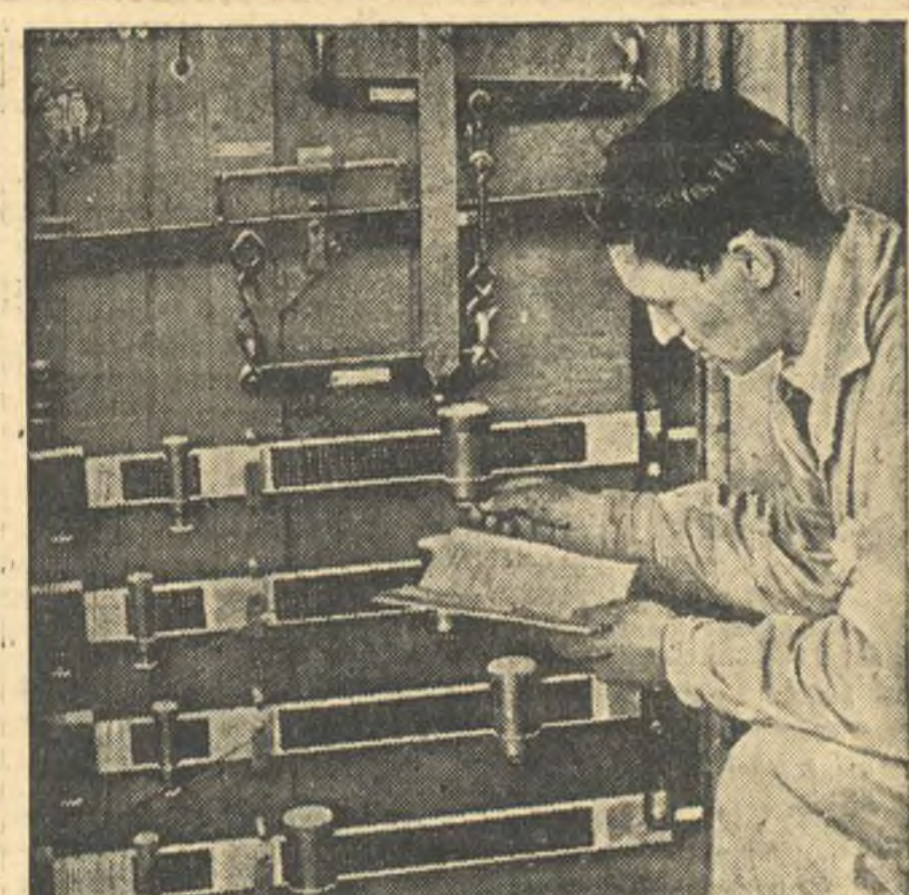
СТРОИТЕЛЬСТВО ДВОРЦА СОВЕТОВ (Москва). Управлением строительства Дворца выстроен специальный бетонный завод, все процессы работы которого механизированы и автоматизированы. Изготовление каждого полутора кубометров бетона на заводе занимает всего три минуты. Отвешивание составных частей бетона занимает 45 секунд. Весь завод обслуживается 10-ю работниками в смену.
