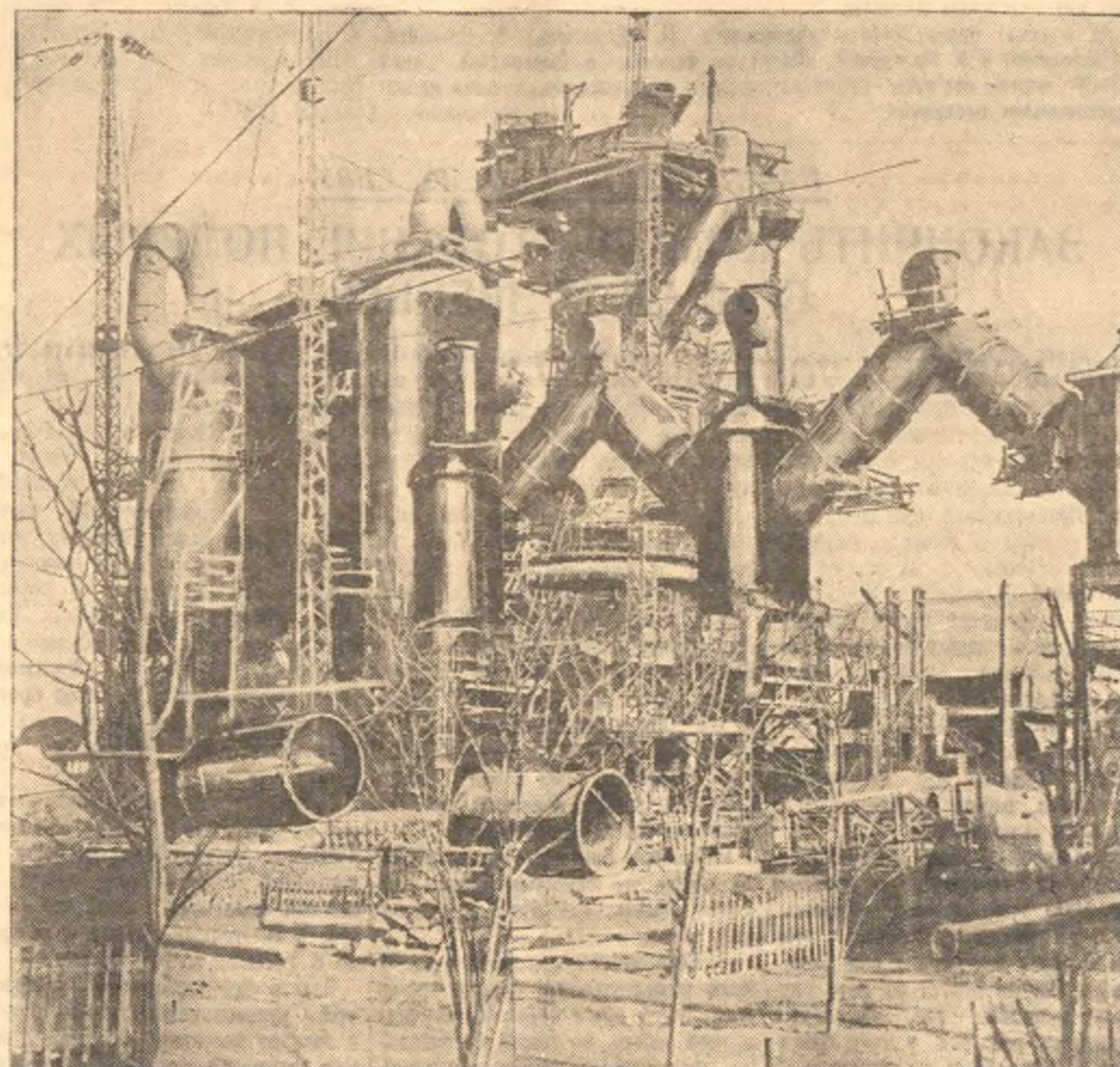
Советская металлургия обогатится в этом году тремя самыми крупными в Европе доменами, которые строятся в Запорожье, Кривом Роге и Мариуполе («Азовсталь»). Объем каждой из новых доменных печей — 1300 куб. метров. На снимке: монтаж новой домы на Криворожском металлургическом заводе. (Соб. фото).
