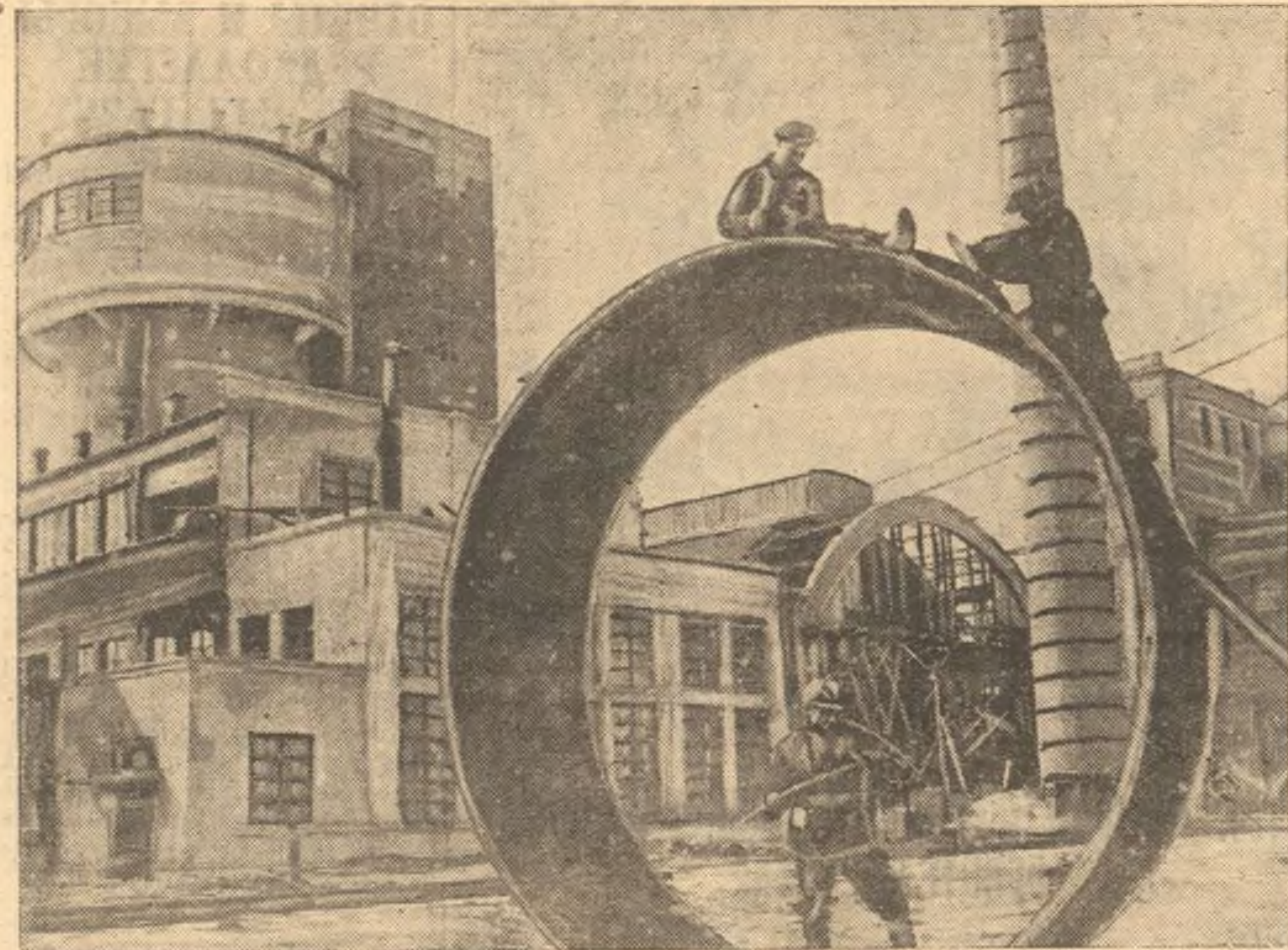
В третьем квартале т. г. будет сдана в эксплуатацию первая очередь Камышинского завода стекольной тары (Сталинградская область). Мощность первой очереди 50 миллионов штук банок в год. На снимке: подготовка кожуха генератора и установке. Слева — вид одного из корпусов завода. (Сокофот).
