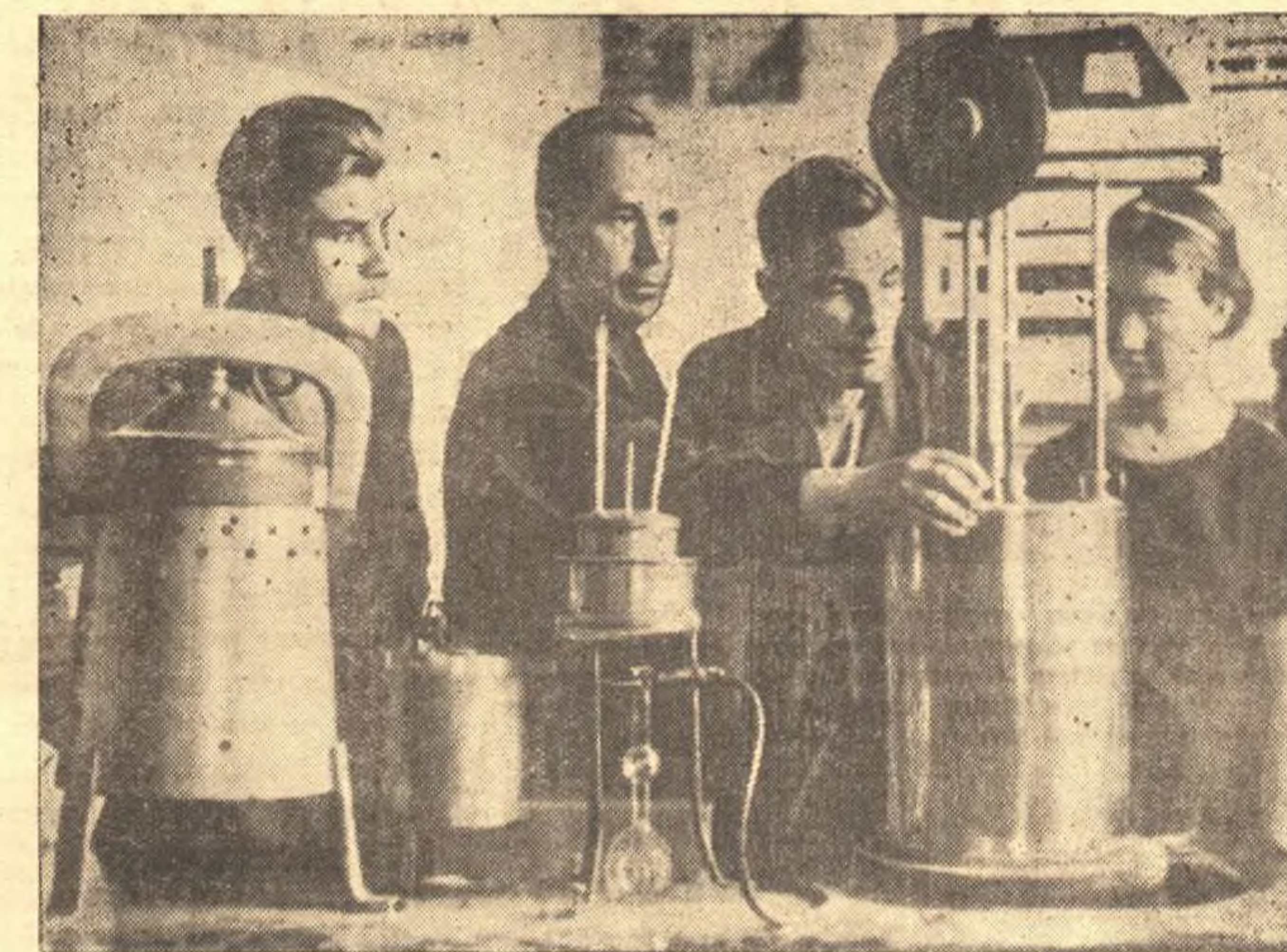
В индустриальном институте для абитуриентов организована техническая выставка. На снимке: доцент Н. И. Норкин (второй слева) знакомит абитуриентов с прибором для определения теплотворной способности топлива (калориметром).
