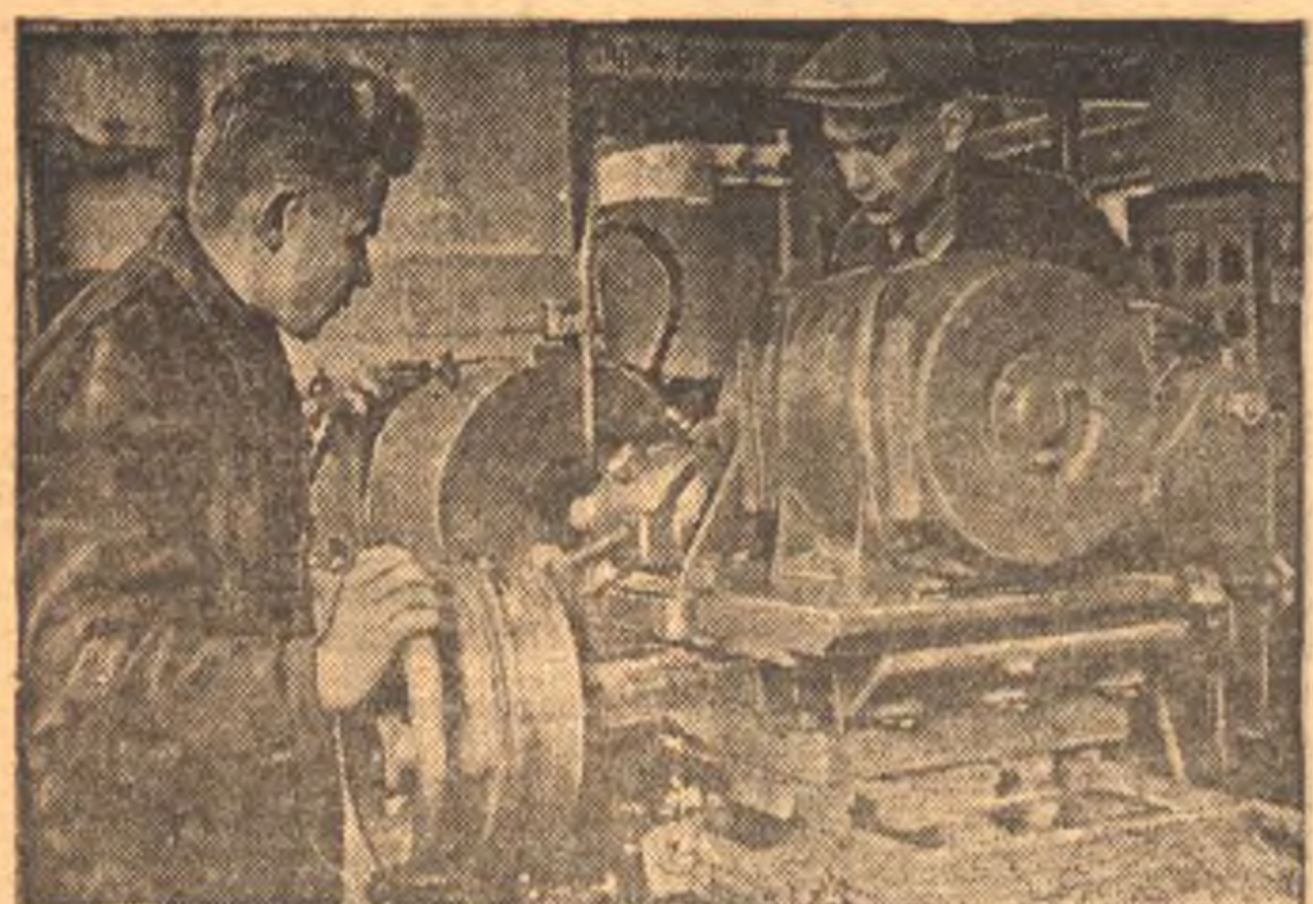
На заводе «Станконормаль» (Москва) заканчиваются внутривзводные испытания универсального внутришлифовального станка «325-Д». В 1940 году завод приступит к серийному выпуску станков «325-Д». На снимке: слесари по сборке И. В. Иванов (слева) и мастер В. И. Алексин — за испытанием станка. (Фото-кино ТАСС).
