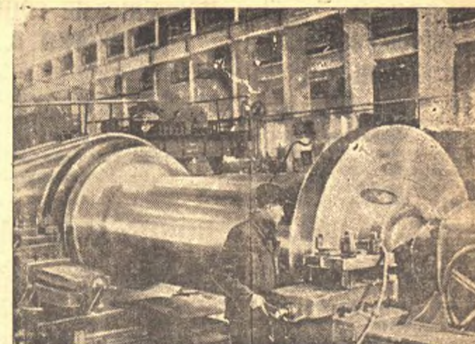
В гидроэлектростанции пехе завода имени Сталина (Ленинград) идет сборка деталей второй гидротурбины для Большой Волги, мощностью в 55 тысяч киловатт. На снимке: токарная обработка промежуточного вала гидротурбины. У станка токаря В. А. Березинский. Фото-клише ТАСС.
