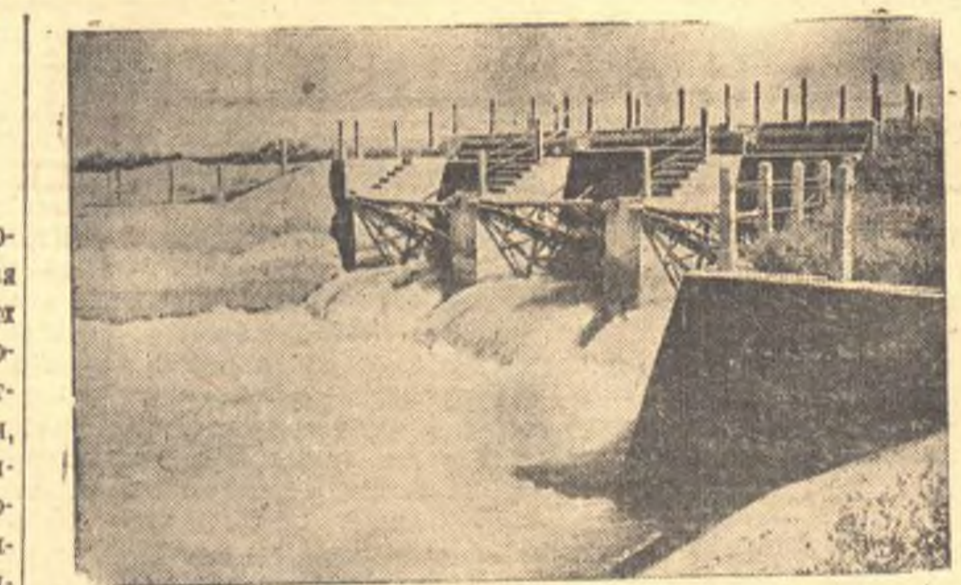
Земли бывшей «Голодной степи» (Южный Казахстан) ныне орошают воды канала имени Кирова. Осваиваются новые посевные площади. На снимке: магистральный канал имени Кирова. Перепад на 59 километре.
