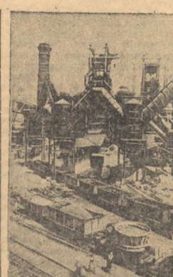
Сталино. На металлургическом заводе имени Сталина трест «Стальинметаллургострой» заканчивает восстановление третьей по счету доменной печи № 1. Работы на домне механизированы и автоматизированы. На снимке: домна № 1 завода имени Сталина. Фотохроника ТАСС.
