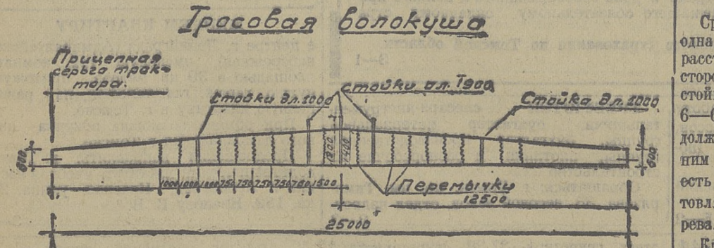
Рис. 1. Общий вид волокуши в растяжку.
