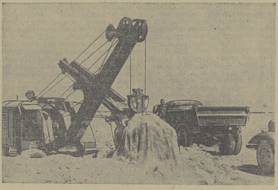
Строительство Главного Туркменского канала. Добыча песка экскаватором в Ходнейминском гравийно-песчаном карьере.
