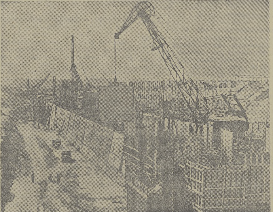
ВОЛГОДОНСТРОИ. По объему выполненных работ коллектив шлоза № 13 идет впереди строителей других сооружений канала. Коллектив шлоза с честью выполняет свои социалистические обязательства. Уже идет установка последних яруса арматуры стенок камеры шлоза, железобетонных плит облицовки и укладки бетона в облицованные участки стенок. На снимке: установка цитов опалубки для бетонирования 2-го яруса верхней головы шлоза № 13. Фотохроника ТАСС.
