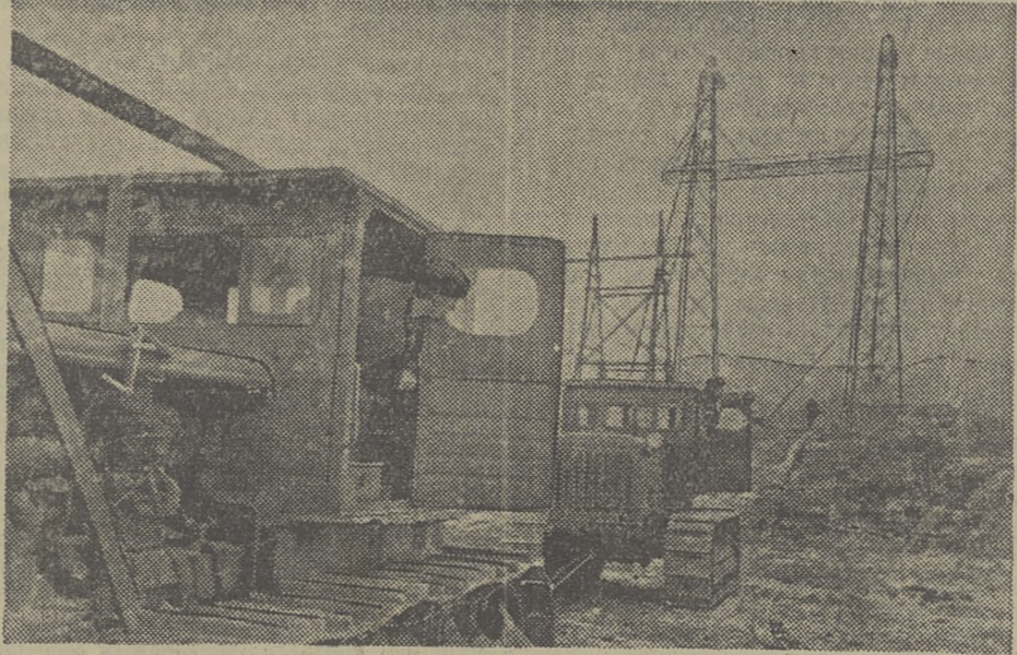
Куйбышевгидрострой. Строители успешно сооружают самый большой в мире воздушный переход высоковольтной линии электропередачи через Волгу. Для подвески тросов воздушного перехода высоковольтной линии строители применили мощные тракторы. На снимке: натяжка тросов линии электропередачи при помощи двух тракторов. (Фотохроника ТАСС).
