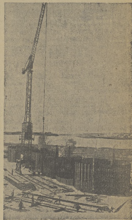
Строительство Каховской гидроэлектростанции. Забивая металлического шпунта в верхнюю перемычку в пойме Днепра.
