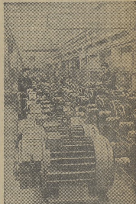
На московском заводе «Динамо» имени С. М. Кирова. На снимке: сборка крановых моторов в машинном цехе. (Фотохроника ТАСС).
