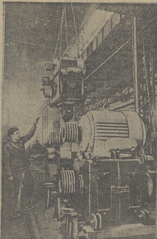
Украинская ССР. Коллектив Днепровского механического завода приступил к выпуску вибраторов «В-104». Новые вибраторы применяются для забивки металлических шпунтов, труб и деревянных свай на строительстве Каховского гидроузла.
