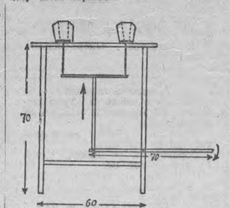
Рис. 1. Поперечный разрез станка простейшего.
