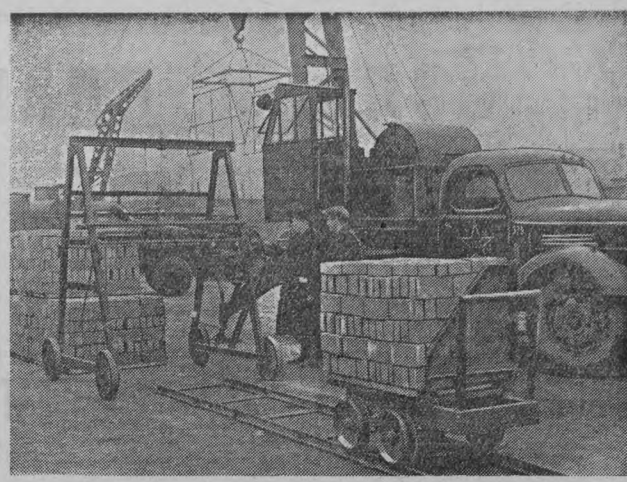
Москва. Лауреат Сталинской премии И. П. Ширков разработал новый способ бесконтейнерной перевозки кирпича в «пакетах». По предложению изобретателя кузов грузовой автомашины оборудован добавочными внутренними бортами, которые со всех сторон крепко сжимают кирпич, уложенный на поддоны. По прибытии машины на строительную площадку с кирпичом при помощи крана быстро выгружаются и подаются на рабочее место каменщика. На снимке: доставка на вагонетках «пакетов» с кирпичом на погрузочную площадку.
