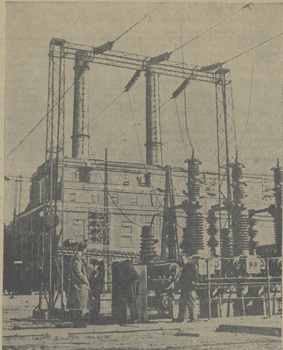
Польская Народная Республика. В Силезии сооружается крупнейшая в стране электростанция «Явожно-П». Строительство этого гиганта польской энергетики ведется при братской помощи Советского Союза. Станция полностью оснащается новейшим советским оборудованием. Введенные в эксплуатацию две первые турбины уже дают ток стране. На снимке: вид электростанции «Явожно-П».
