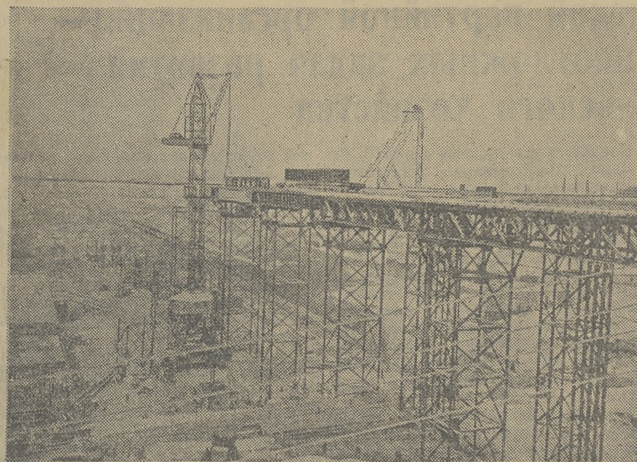
Куйбышевгидрострой. Над котлованом для здания гидроэлектростанции на высоте 40 метров сооружается бетонная эстакада. На ней монтируются стальные пути, по которым будут двигаться порталы кранов и мотовозы, доставляющие в котлован бетон, арматуру и различное оборудование. На снимке: строительство бетонной эстакады. (Фотохроника ТАСС).
