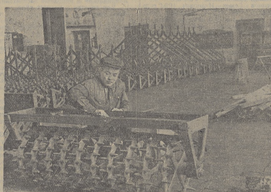
Курган. Для обработки почвы по новой системе, предложенной директором Шадринской опытной станции Т. С. Малышевым, применяются кольчатые катки, которые выпускает курганский завод «Уральский». Уже выпущено более 1.800 катков. До конца года будет выпущено еще около 200 катков. На снимке: слесарь В. Г. Ломов за сборкой кольчатых катков. (Фотохроника ТАСС).
