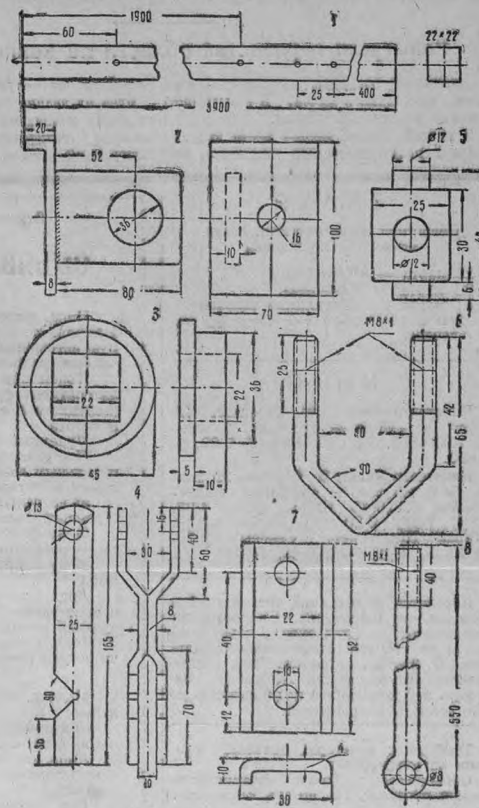
Рис. 8. Детали механизма управления. 1. Квадратный вал, 1 штука; 2. Корпус подшипника, 3 штуки; 3. Подшипник, 3 штуки; 4. Короткий поводок квадратного вала, 6 штук; 5. Сухарь, 7 штук; 6. Скоба, 7 штук; 7. Пластина, 7 штук; 8. Тяга узлоуловителя, 1 штука.
