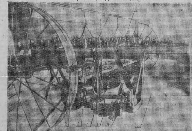
Рис. 1. Переоборудованная сеялка СД-24 для посева кукурузы квадратно-гнездовым способом. 1. Узлоуловитель; 2. Квадратный вал; 3. Длинный поводок квадратного вала; 4. Тяга узлоуловителя; 5. Кронштейн узлоуловителя; 6. Мерная проволока; 7. Короткий поводок квадратного вала; 8. Пружина.
