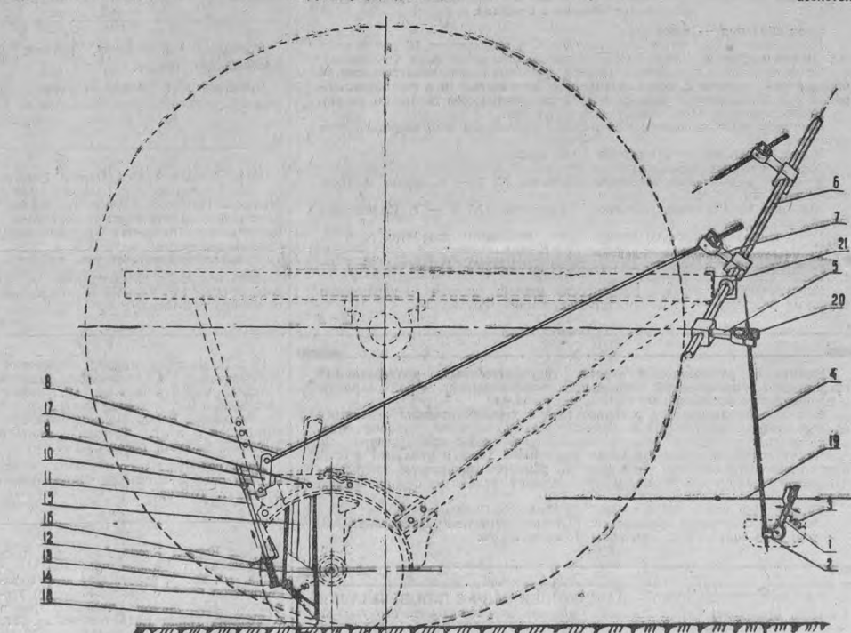
Рис. 2. Общая кинематическая схема привода клапанов. 1. Вилка узлоуловителя; 2. Рычаг вилки узлоуловителя; 3. Пружина узлоуловителя; 4. Тяга узлоуловителя; 5. Длинный поводок квадратного вала; 6. Квадратный вал; 7. Короткий поводок квадратного вала; 8. Тяга; 9. Рычаг; 10. Сухарь; 11. Тяга клапана; 12. Пружина клапана; 13. Ось клапана; 14. Клапан; 15. Труба накопителя; 16. Упор пружины клапана; 17. Стопорный болт; 18. Чистик; 19. Мерная проволока; 20. Сухарь; 21. Подшипник.
