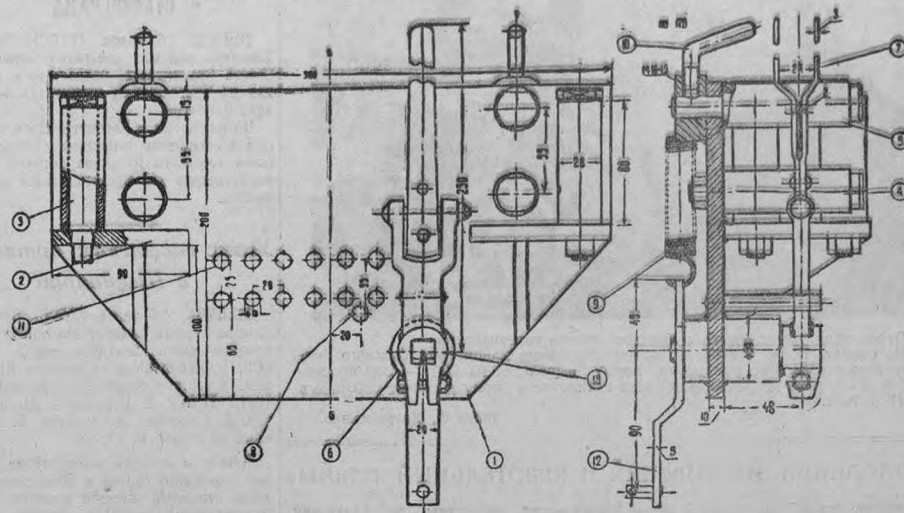
Рис. 3. Чертеж упрощенной конструкции узлоуловителя. 1. Пластина; 2. Подшипник; 3. Вертикальные ролики; 4. Горизонтальные ролики; 5. Съемные ролики; 6. Вилка узлоуловителя; 8. Упор; 9. Пружина; 10. Стопорный болт; 11. Отверстия для крепления и регулировки узлоуловителя; 12. Поводок; 13. Валок.
