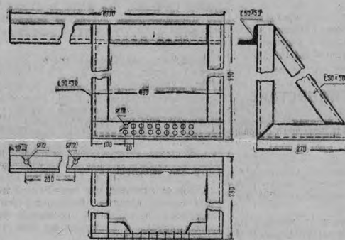
Рис. 5. Кронштейн узлоуловителя.
