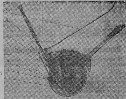
Рис. 6. Накопитель зерна с клапаном. 1. Клапан; 2. Труба накопителя; 3. Пружина клапана; 4. Упор пружины клапана; 5. Тяга клапана; 6. Сухарь; 7. Ось рычага клапана; 8. Рычаг; 9. Тяга.
