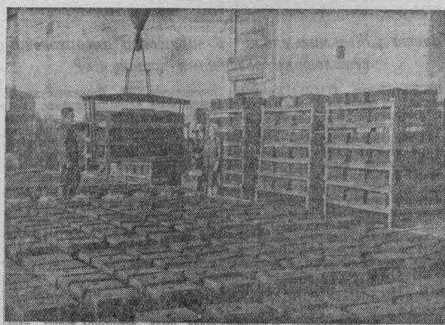
В литейном цехе томского электромеханического завода имени В. В. Вахрушева применяется новый этаперный способ расстановки безопычных форм перед заливкой. Применение нового способа дает возможность ставить дополнительно около 700 форм без расширения производственной площади.
