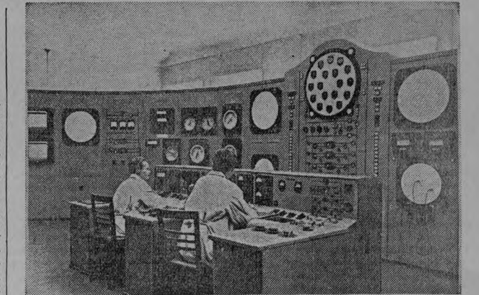
Первая советская атомная электростанция Академии наук СССР. На снимке: главный пункт управления.
