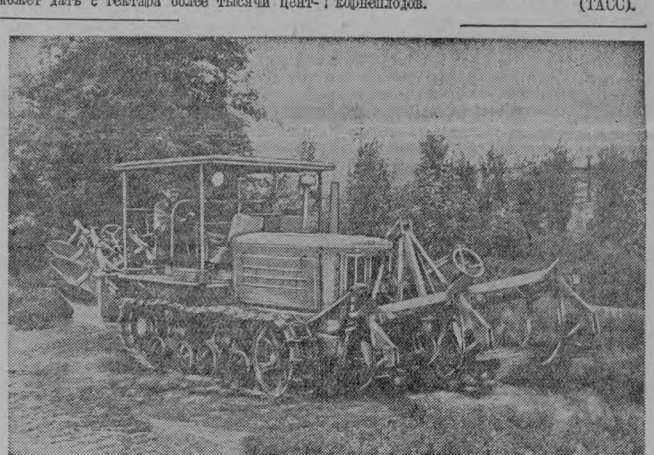
Сталинградский тракторный завод выпустил опытный трактор «ДТ-57 круглосклонный», предназначенный для освоения земель в горных районах страны. Он может производить вспашку земли на крутых склонах гор, двигаться вперед и назад без поворотов, с одинаковыми скоростями (работать «сцепным» способом). Отличие его от трактора «ДТ-54» состоит в том, что он производит работу навесными орудиями, расположенными спереди и сзади.
