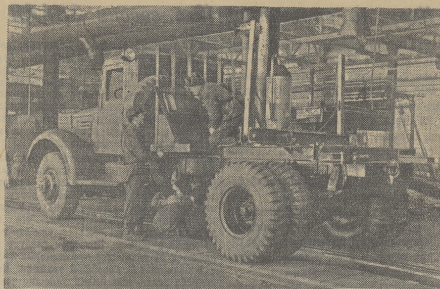
Белорусская ССР. Минский автозавод на базе автомашины МАЗ-200 создал новый лесовоз. Он оснащен двумя ведущими мостами, обладает высокой проходимостью в условиях лесной и заболоченной местности. Лесовоз, снабженный прицепом, предназначается для транспортировки древесины. Общая грузоподъемность его с прицепом составляет 15 тонн. С помощью прицепа лесовоз может перевозить хлысты длиной до 30 метров. На снимке: новый лесовоз на отделочном конвейере цеха сборки и испытания автомобилей.
