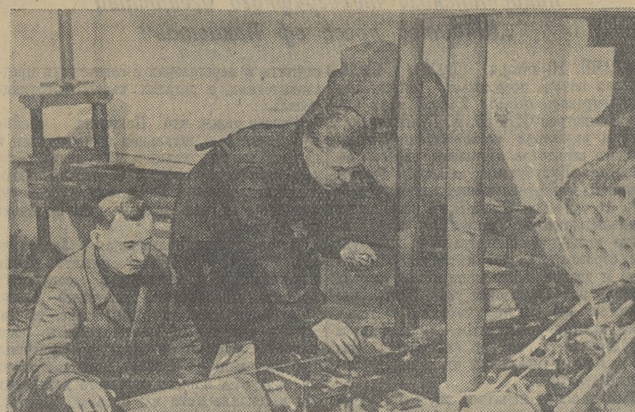
Кафедра горных машин и рудничного транспорта политехнического института. У стенда для испытания пневматических буровых молотков — аспирант И. Басов (справа) и учебный мастер Э. Лисовский.
