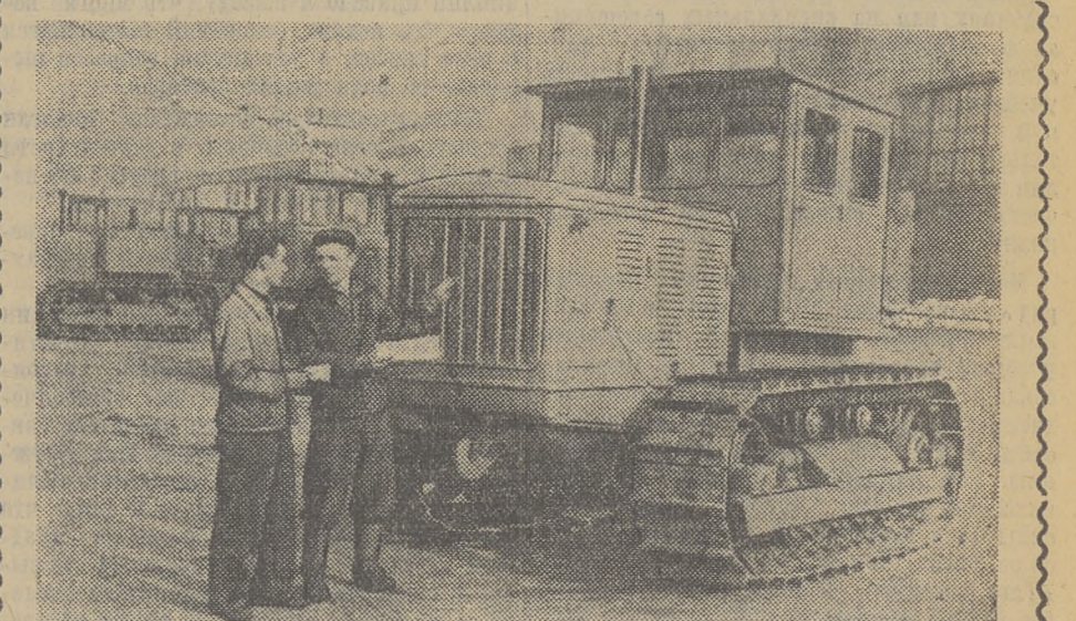
Челябинский тракторный завод начал выпуск опытной партии новых стальных тракторов «С-100». Этот трактор имеет более совершенную систему смазки подшипников коленчатого вала, поршней, улучшенный процесс газораспределения и поддона топлина, выданные повышенного качества, хорошие устройство и подкачки топлива и некоторые другие усовершенствования.
