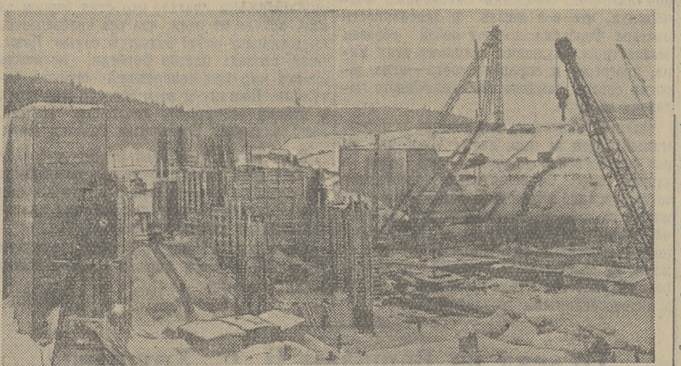
На строительстве Уфимской ГЭС уже обрисовались контуры будущего плота. Сейчас здесь идут работы по установке арматуры и укладке бетона. На снимке: нижняя голова плотины Уфимской ГЭС. (Фотохроника ТАСС).
