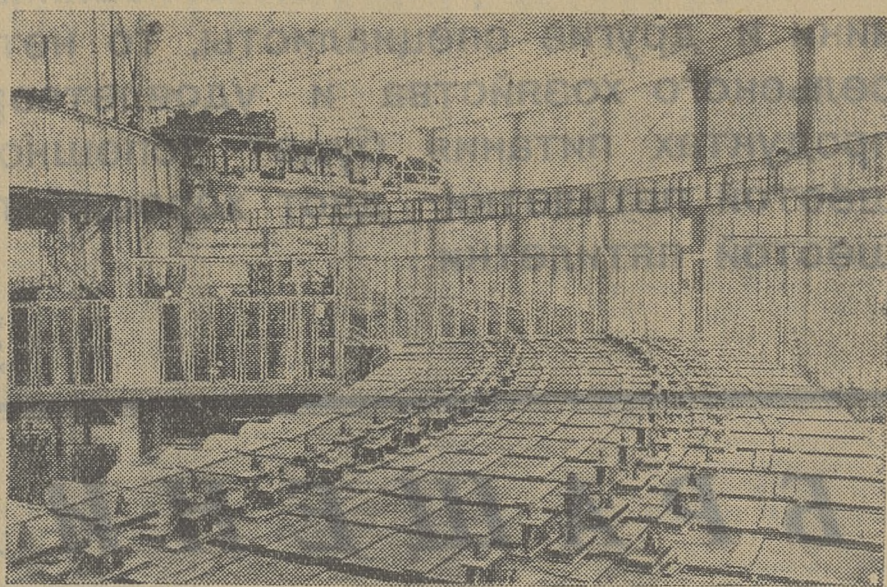
В электрофизической лаборатории Академии наук СССР создана гигантская установка для изучения атомного ядра. Сейчас заканчивается монтаж и ведутся работы по наладке самого мощного в мире синхротрона, с помощью которого ученые ускорят протоны до энергии в десять миллиардов электронов. Кольцевой электромагнит нового ускорителя весит 36 тысяч тонн, его диаметр достигает почти 60 метров. Новый ускоритель даст возможность изучать ядерные процессы при сверхвысоких энергиях. На снимке: часть электромагнита синхротрона (вид сверху). (Фотохроника ТАСС).
