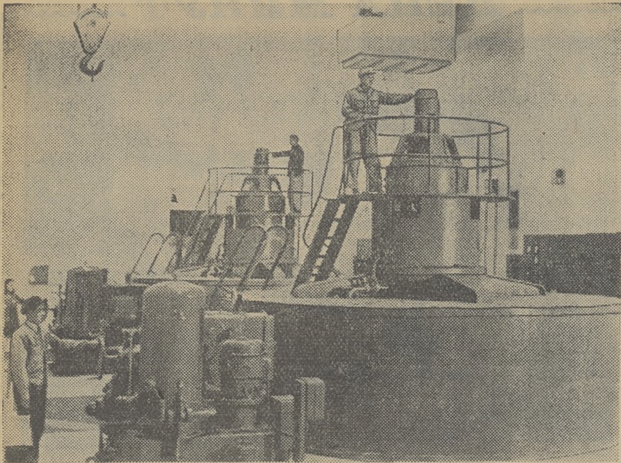
Китайская Народная Республика. В Гуяне (провинция Фунзянь) вступила в строй новая гидроэлектростанция. Она построена по проекту китайских инженеров и оборудована генераторами отечественного производства. На снимке: гидротурбинные генераторы электростанции. (Фотохроника ТАСС).
