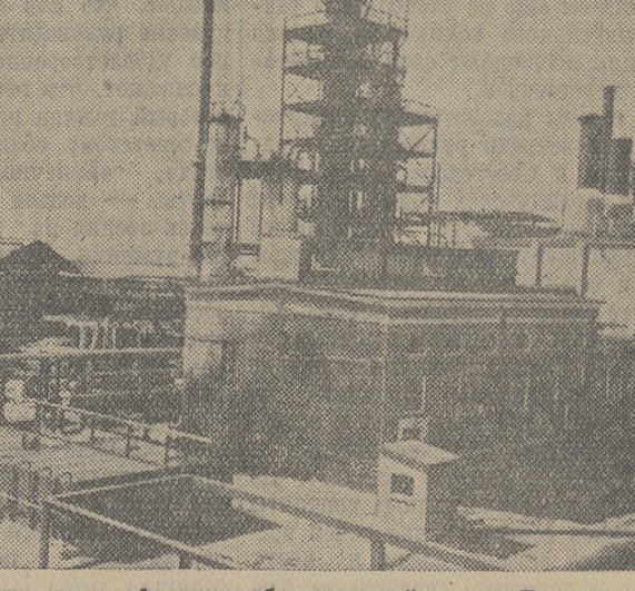
В Омске сооружается нефтеперерабатывающий завод. В конце апреля дали промышленную продукцию крекинг-установки, предназначенные для получения высокооктановых сортов бензина и керосина из мауэта. Все механизмы работают хорошо. Апрельский план завод перевыполнил. На снимке: общий вид крекинг-установки. (Фотохроника ТАСС).
