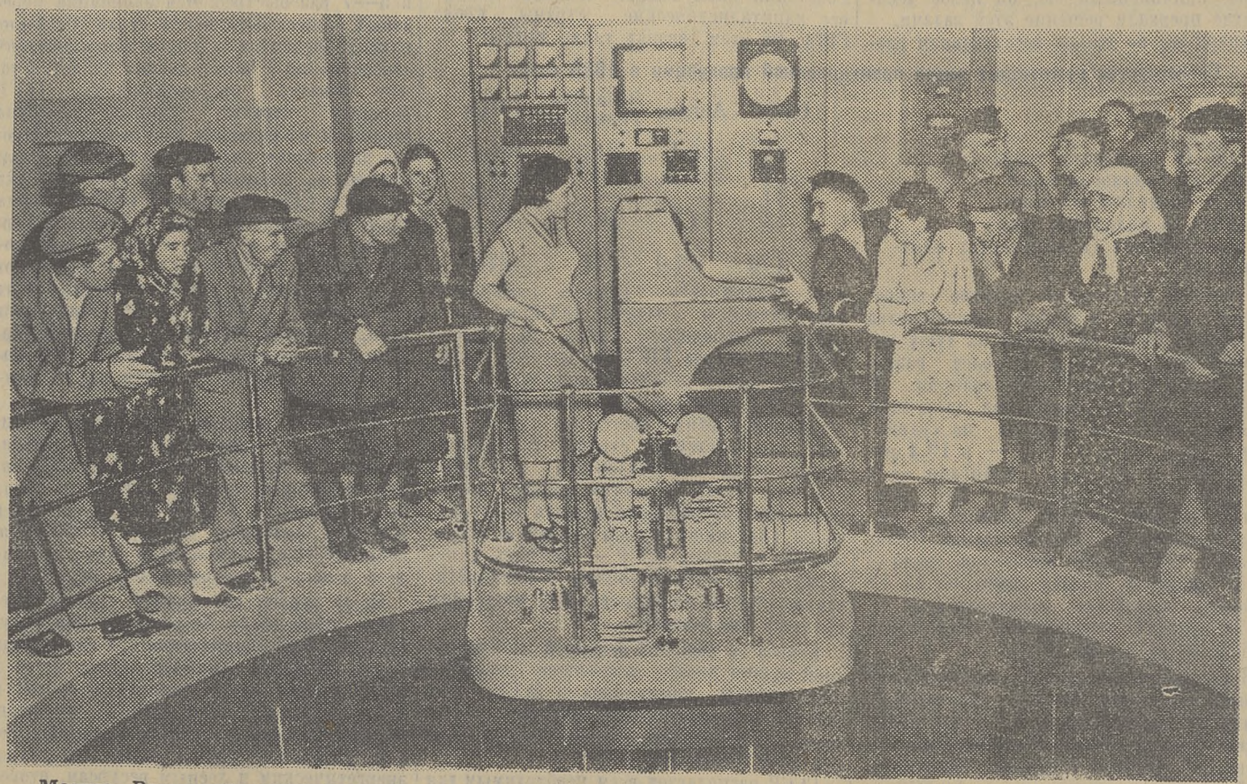
Москва. Всесоюзная промышленная выставка 1956 года. На снимке: посетители в павильоне «Атомная энергия в мирных целях» осматривают действующий атомный реактор. (Фотохроника ТАСС).
