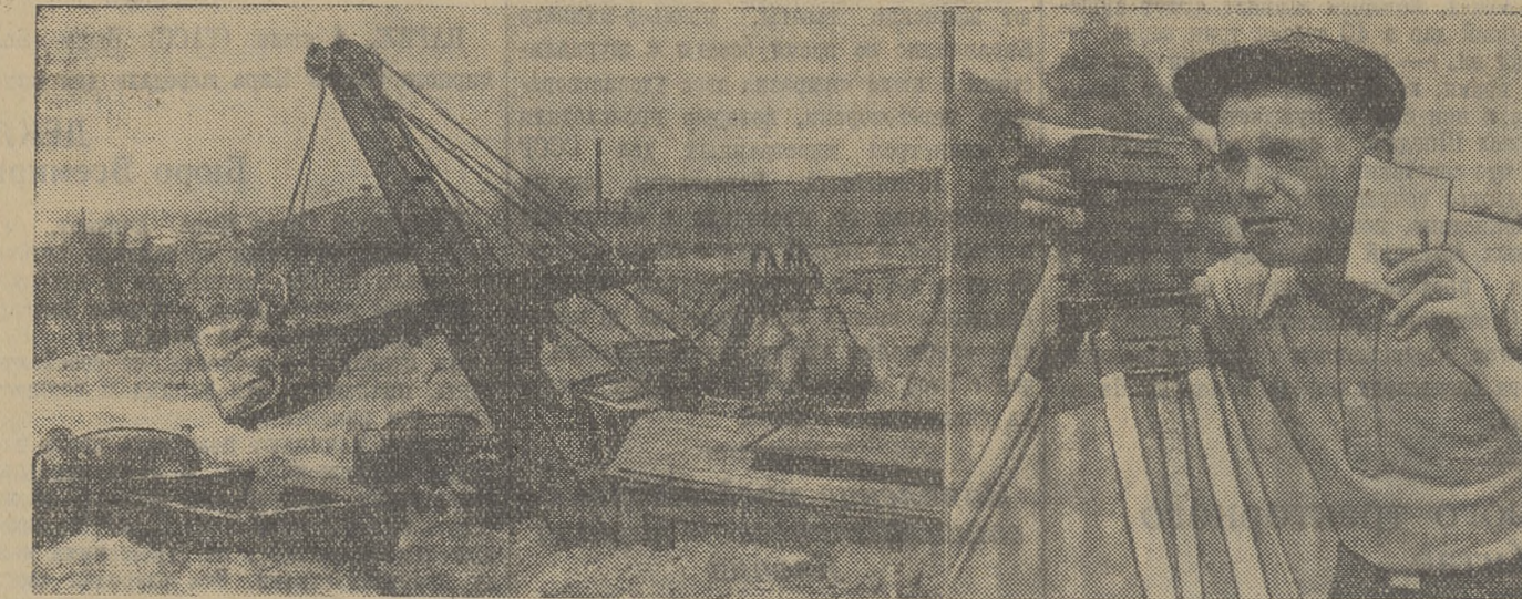
В Томске ведется строительство второй очереди трамвайного пути. На снимках: 1. Земляные работы на Дальне-Ключевской улице. 2. Инженер конторы «Облпроект» Д. И. Кологривов ведет вертикальную съемку местности.
