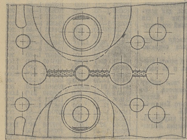
Рис. 1. Эскиз расположения центральной щели в антидетонационной головке двигателя ТМА.
