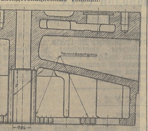
Рис. 2. Эскиз поперечного разреза антидетонационной головки двигателя ТМА по расположению центральной щели.
