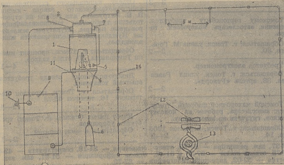
Схема «электропастуха».
