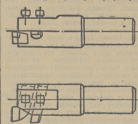
Фиг. 2. Предложенная т. Угрюмовым резцовая установка.
