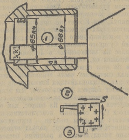
Фиг. 1. Установка трех резцов по старому технологическому процессу.
