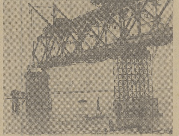
Китайская Народная Республика. Через реку Янцзы в Ухани сооружается большой мост. Он будет иметь девять пролетов. Общая протяженность составит 1 километр 440 метров. По мосту будут проведены железнодорожные линии и автомобильные.
