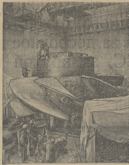
На строительстве Иркутской ГЭС широко развернулось социалистическое соревнование за достойную встречу 39-й годовщины Великого Октября. По плану идет монтаж первого гидроагрегата. Бригада тов. Шайкина ведет сборку рабочего колеса турбины. На снимке бригада тов. Шайкина за монтажом рабочего колеса. (Фотохроника ТАСС).
