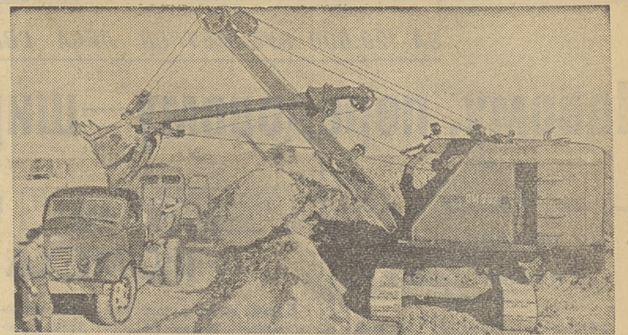
Казахская ССР. На строительстве Карагандинского металлургического завода готовится площадка под доменный пех и роется котлован под коксохимические батареи. Экскаваторы Егора Лапенкова, Григория Гимбарова, Николая Раутцева и других погружали в самосвалы около 400 тысяч кубометров грунта. Десятки передовых механизаторов завершили уже годовые задания. На снимке: подготовка площадки под доменный пех. (Фотохроника ТАСС).
