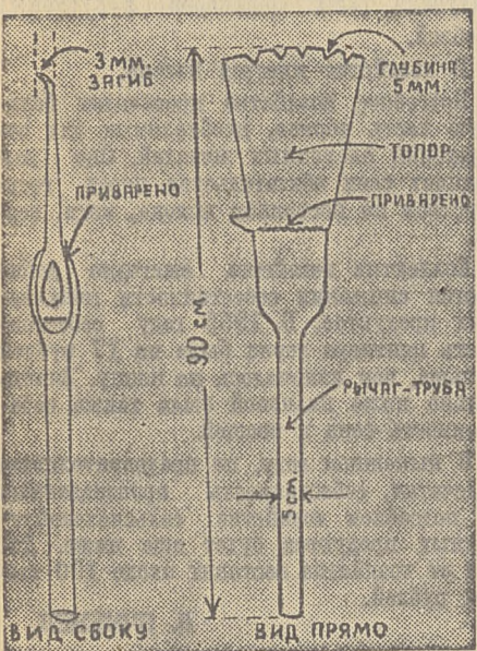
Схема устройства валочного клина.
