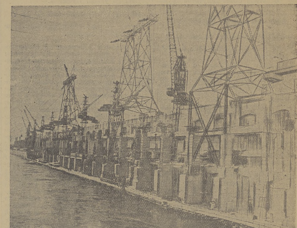
Общий вид здания Куйбышевской ГЭС со стороны верхнего бьефа. (Фотохроника ТАСС).
