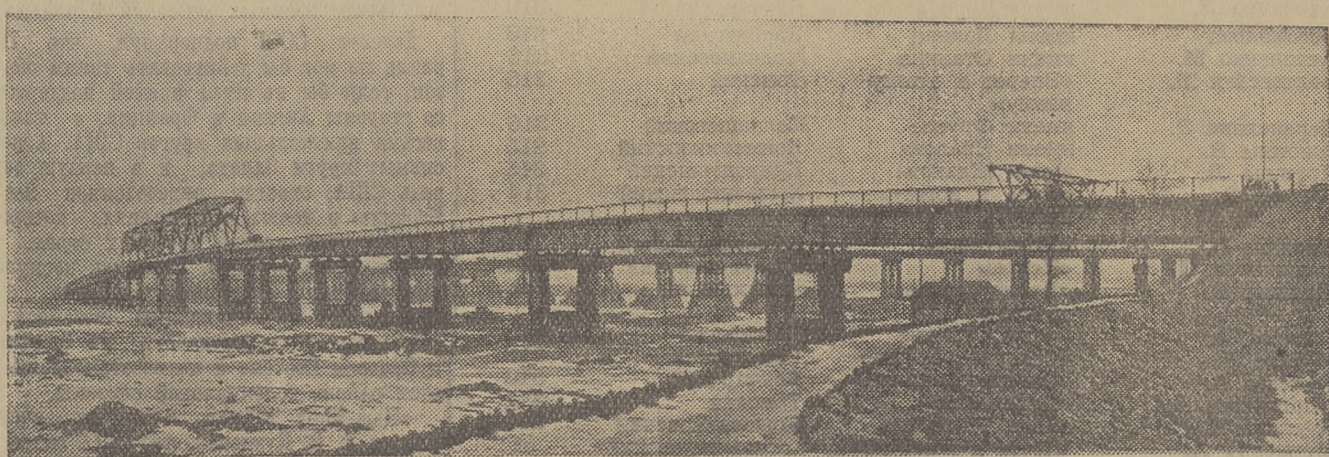
Черныгов. Закончено строительство нового моста длиной 575 метров через реку Десна. При сооружении моста были применены блонн из предварительного напряженного железобетона. Длина каждого блока — 33 метра. На снимке: общий вид нового моста.
