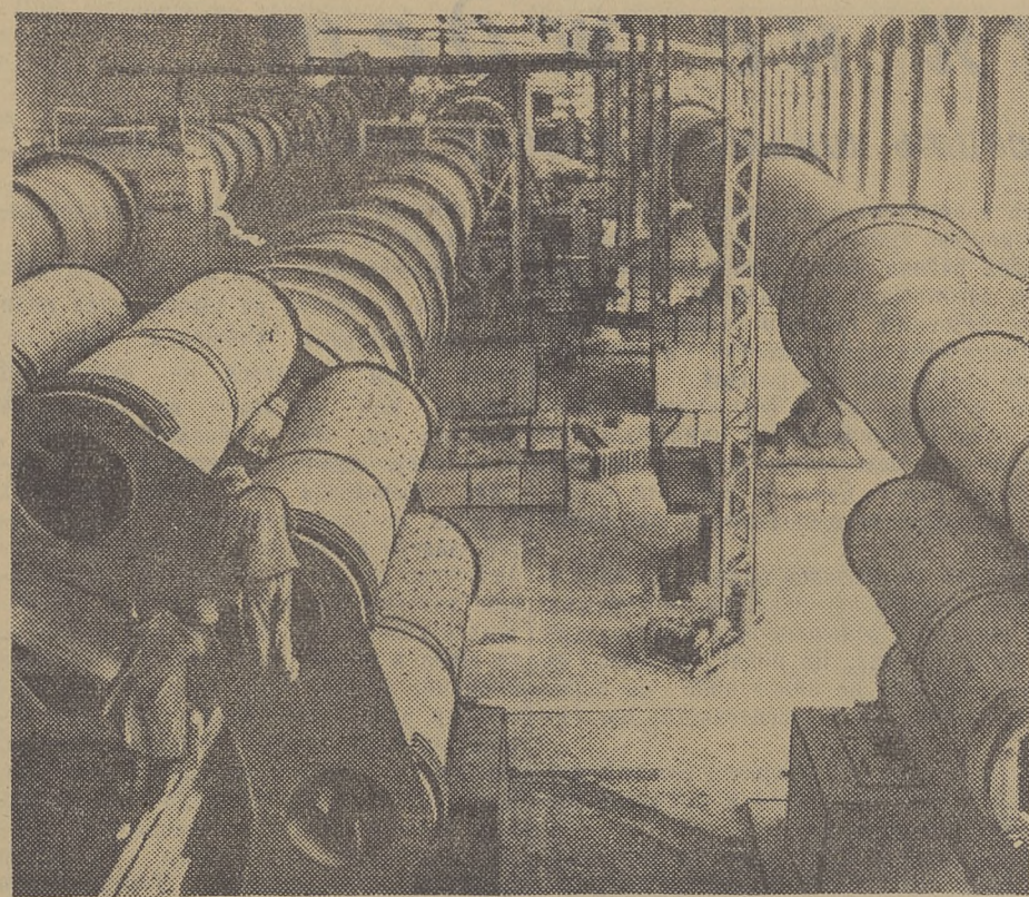
Иркутская область. На окраине города Ангарска сооружается один из крупнейших в стране цементных заводов, который будет дан в эксплуатацию в 40-й годовщину Великого Октября. Уже смонтированы три 150-метровые печи. Началось бетонирование силовых оснований.
