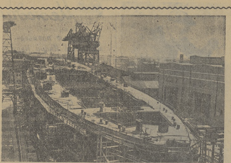
В Ленинграде на судостроительном заводе сооружается атомный ледокол «Ленин».
